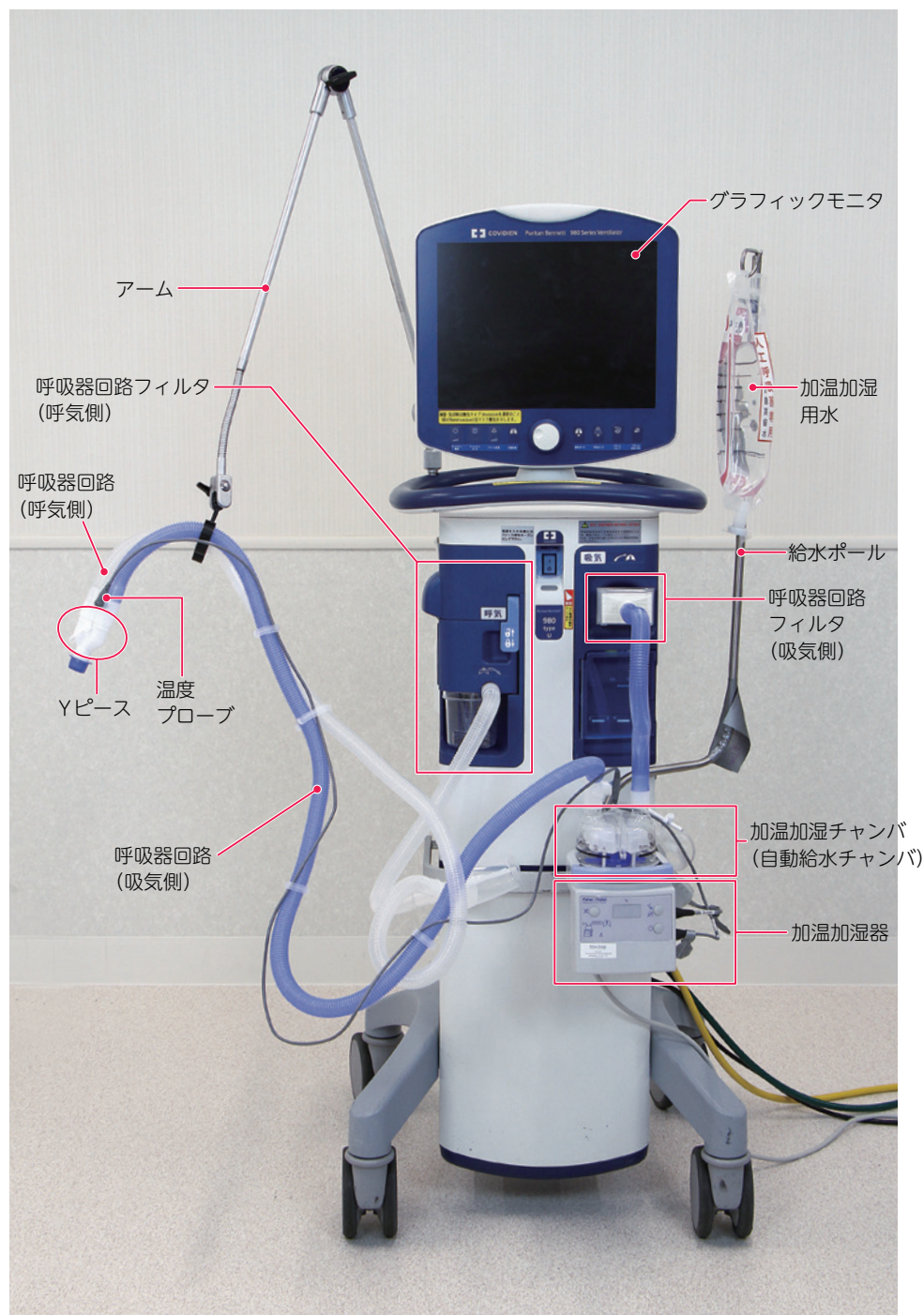
完成した全体像【Puritan Bennett 980】
